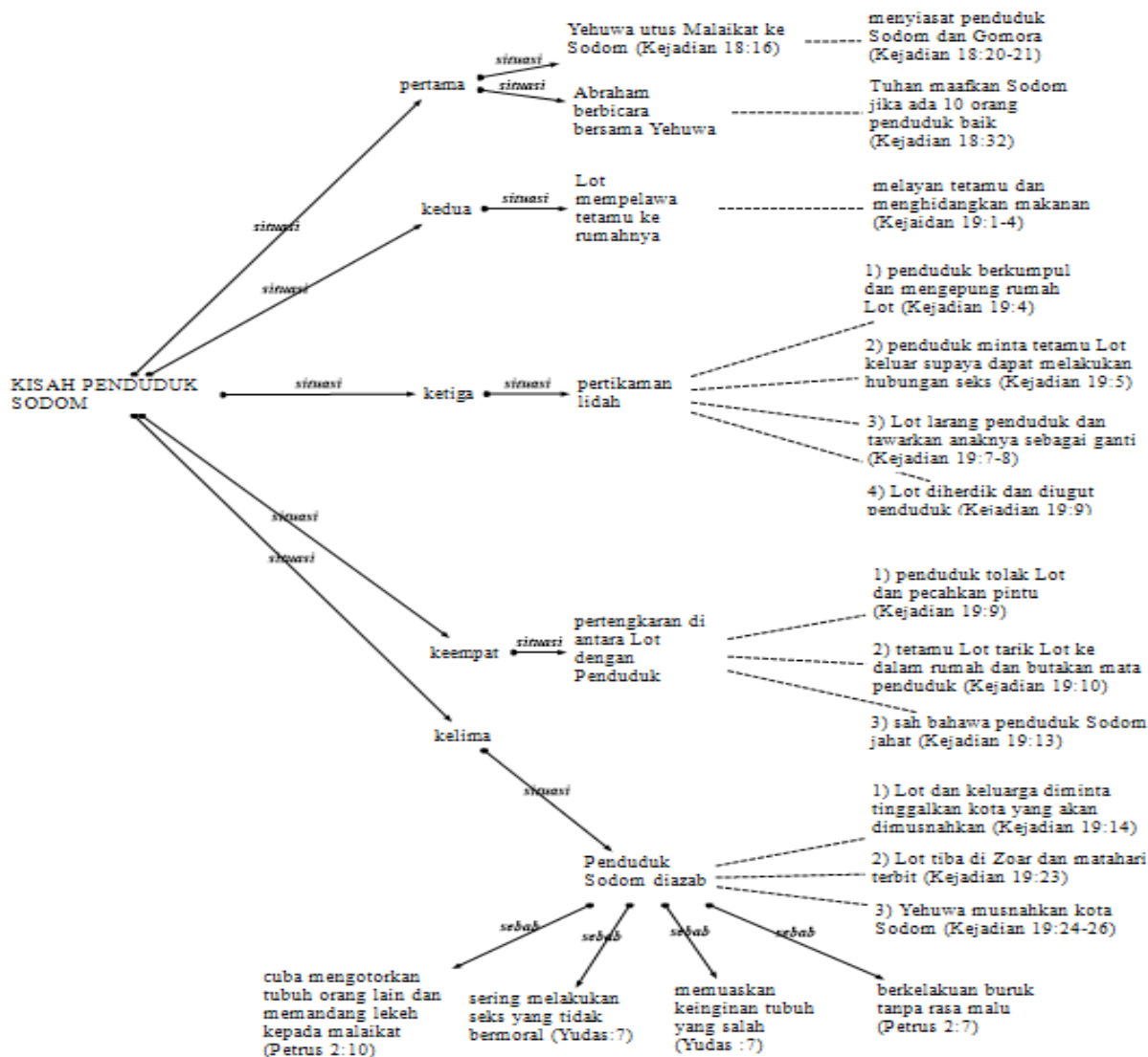
Rajah 3.1: Kerangka Teks Kisah Sodom Menurut Perspektif Bible
