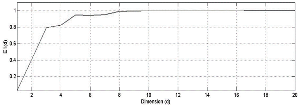
Figure 5. Embedding dimension, E1(d)
